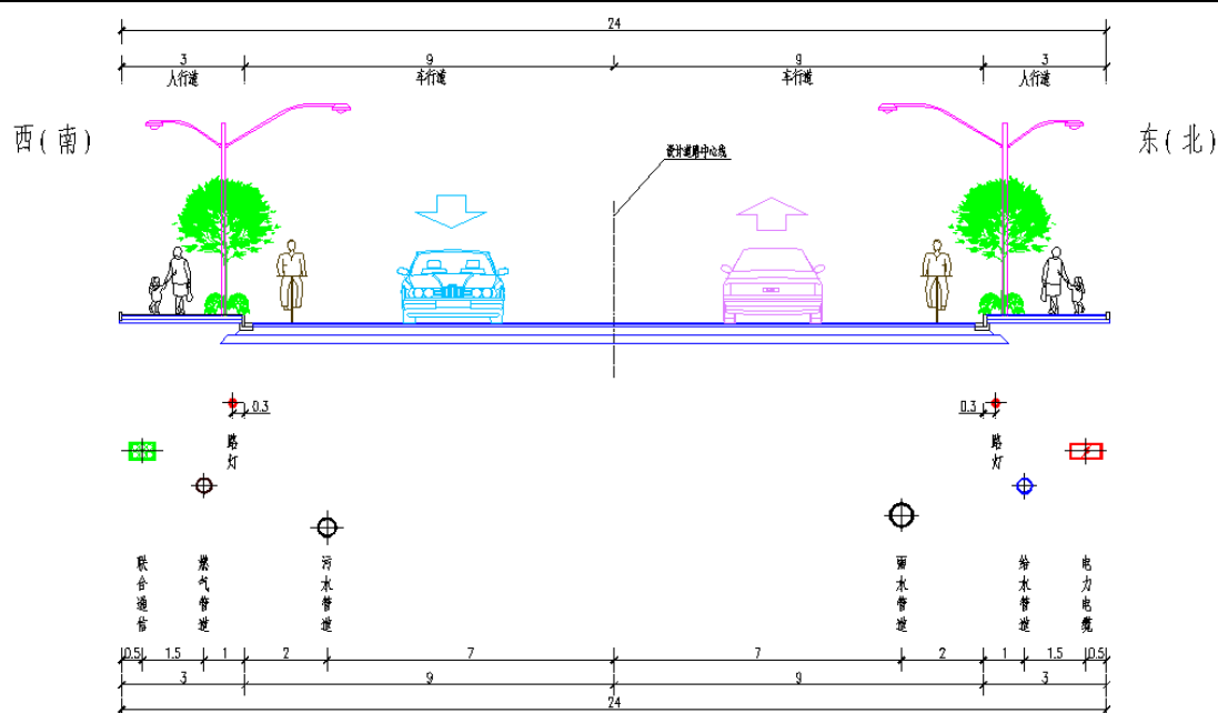
图 1-2 中环路管线综合标准横断面
