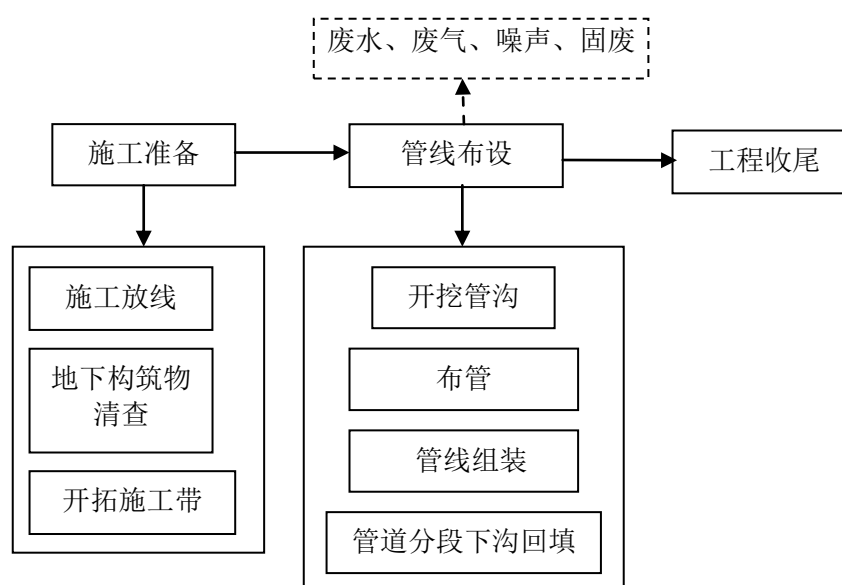
图 5-2 管网敷设工艺流程与产污环节图
