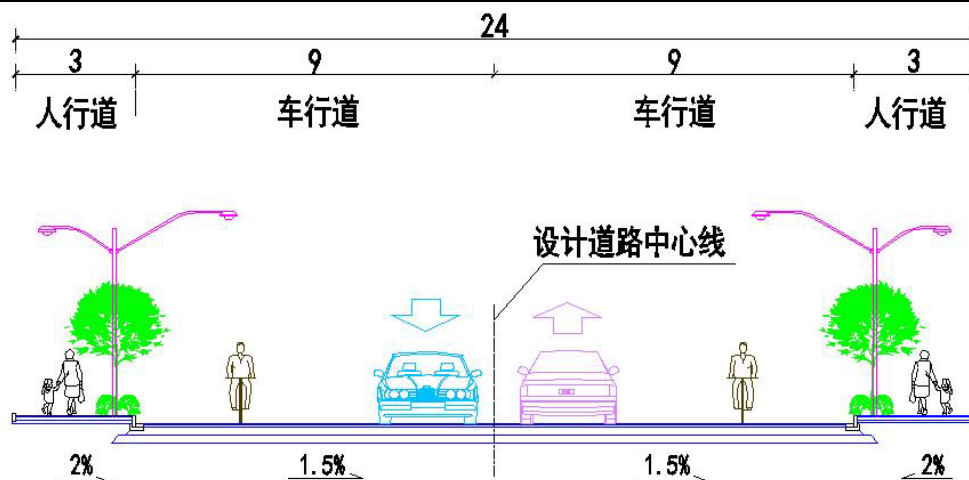
图 1-1 道路标准横断面图
