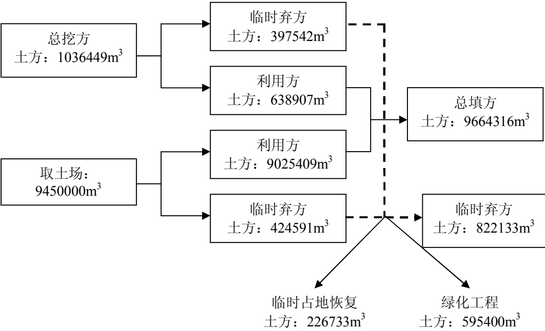
图 2.4-4 拟建项目路基工程土石方平衡图
