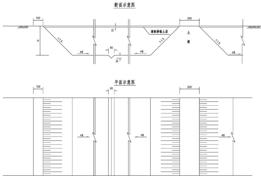
图 4.6-1 鱼塘型取土坑断面与平面图
