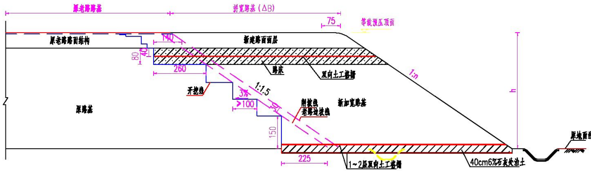
图 2.4-3 路基拼接处理图
