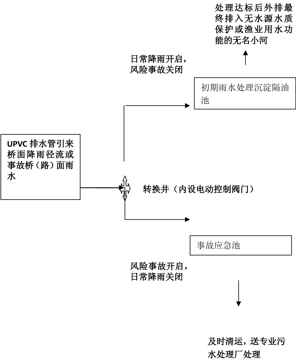
图 6.3-1 初期雨水与事故池处理工艺流程示意图
