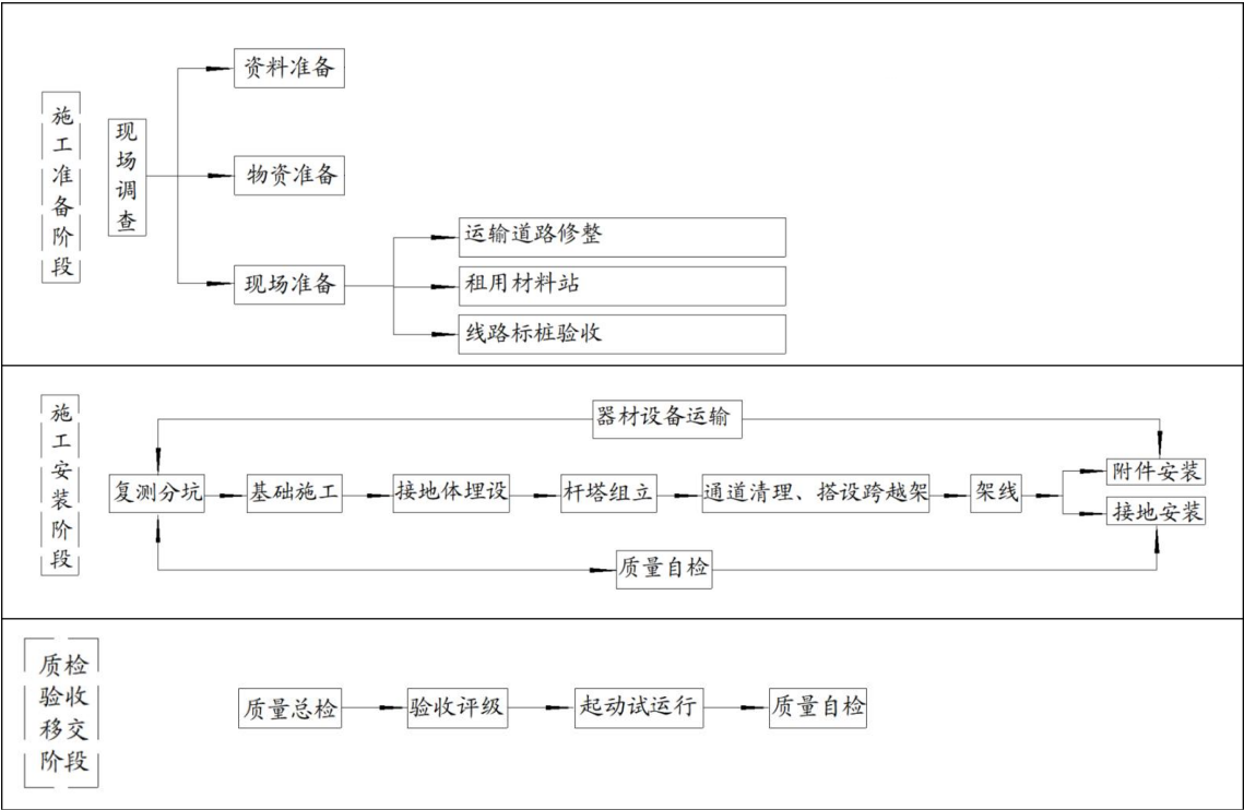
图 3.1-5 新建架空线路施工工艺流程图
