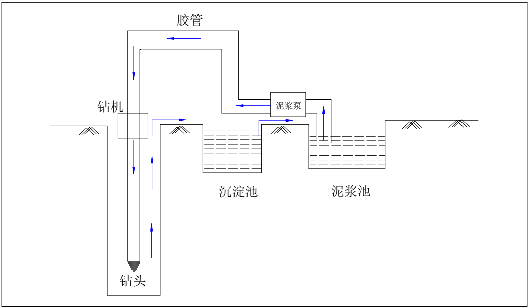
图 3.1-8 采用泥浆护壁钻机反循环法钻进施工工艺
