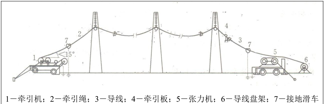
图 3.1-11 牵、张系统构成示意图
