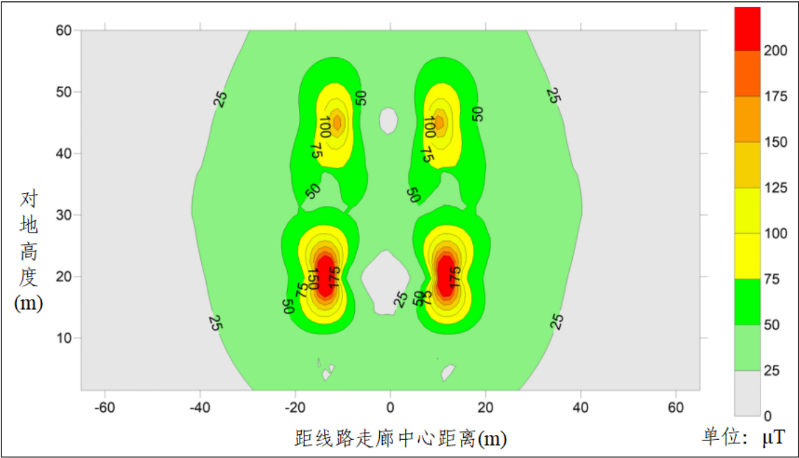
图 6.1-7 恢复架线段 500kV 同塔双回线路 100 \mu\text{T} 等值线分布图
