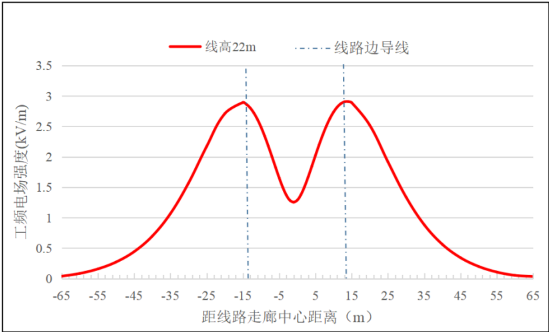
图 6.1-4 新建段 500kV 同塔双回线路工频电场强度分布曲线图
