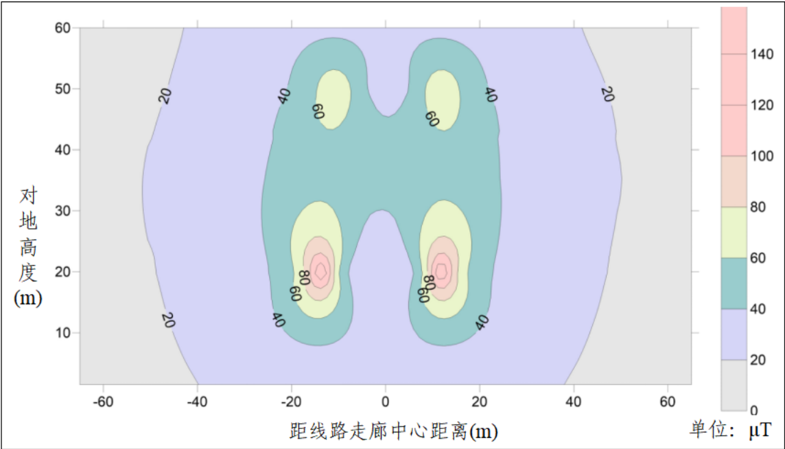
图 6.1-9 新建段 500kV 同塔双回线路 100 \mu T 等值线分布图
