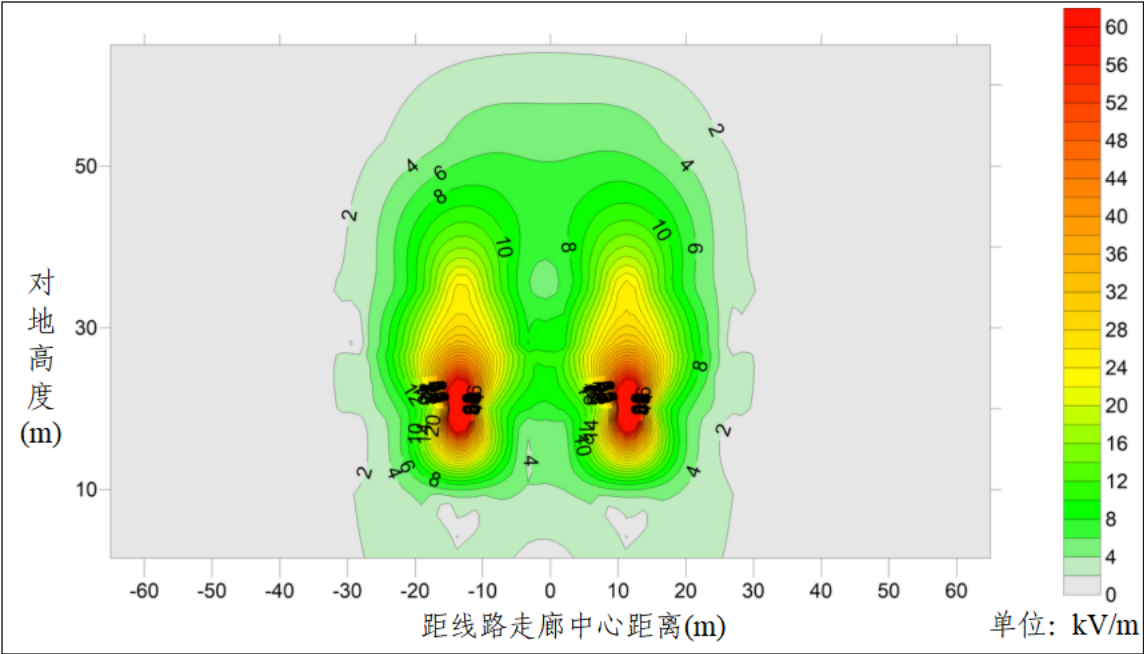
图 6.1-6 恢复架线段 500kV 同塔双回线路 4kV/m 等值线分布图
