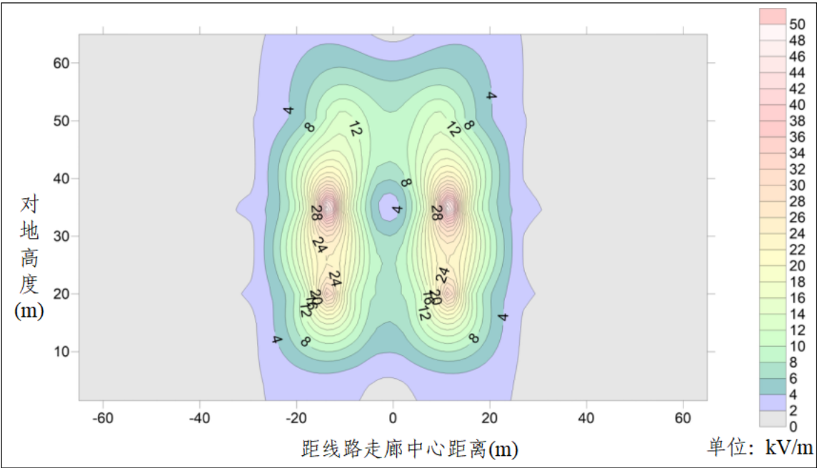
图 6.1-8 新建段 500kV 同塔双回线路 4 \text{kV/m} 等值线分布图
