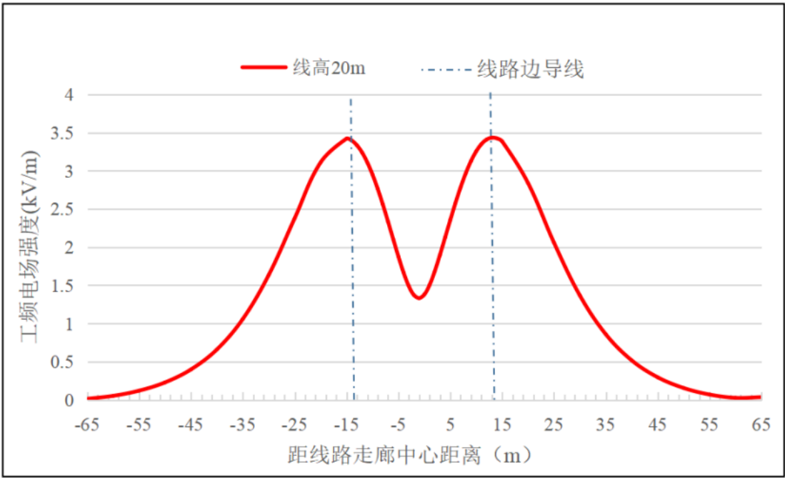
图 6.1-2 恢复架线段 500kV 同塔双回线路工频电场强度分布曲线图
