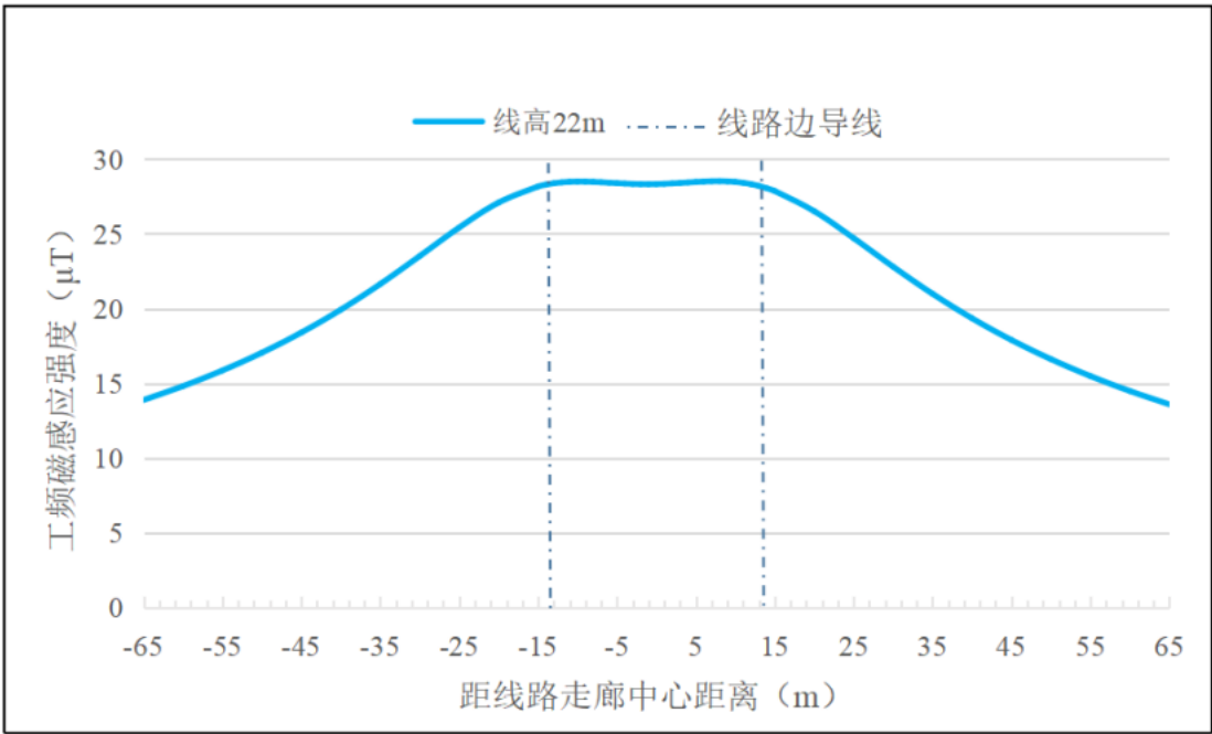
图 6.1-5 新建段 500kV 同塔双回线路工频磁感应强度分布曲线图
