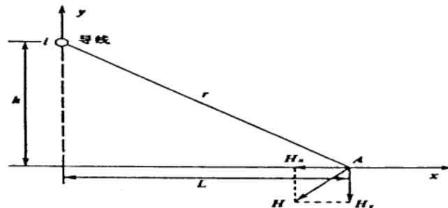
图6.1-1 磁场向量图
