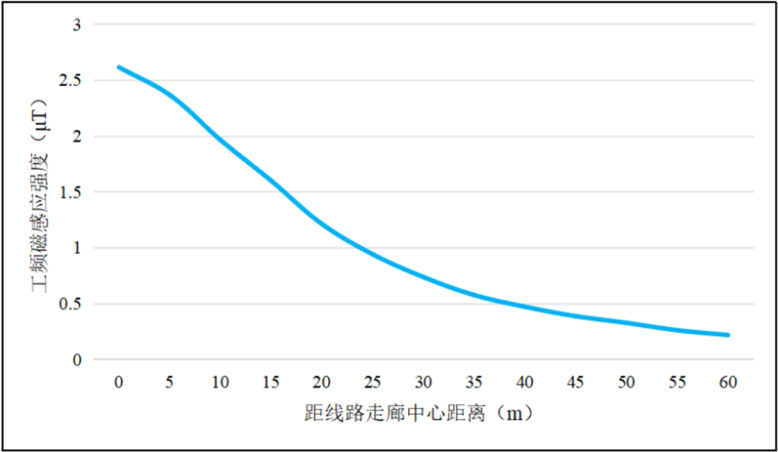
图 6.1-2 类比线路工频磁感应强度变化趋势示意图
