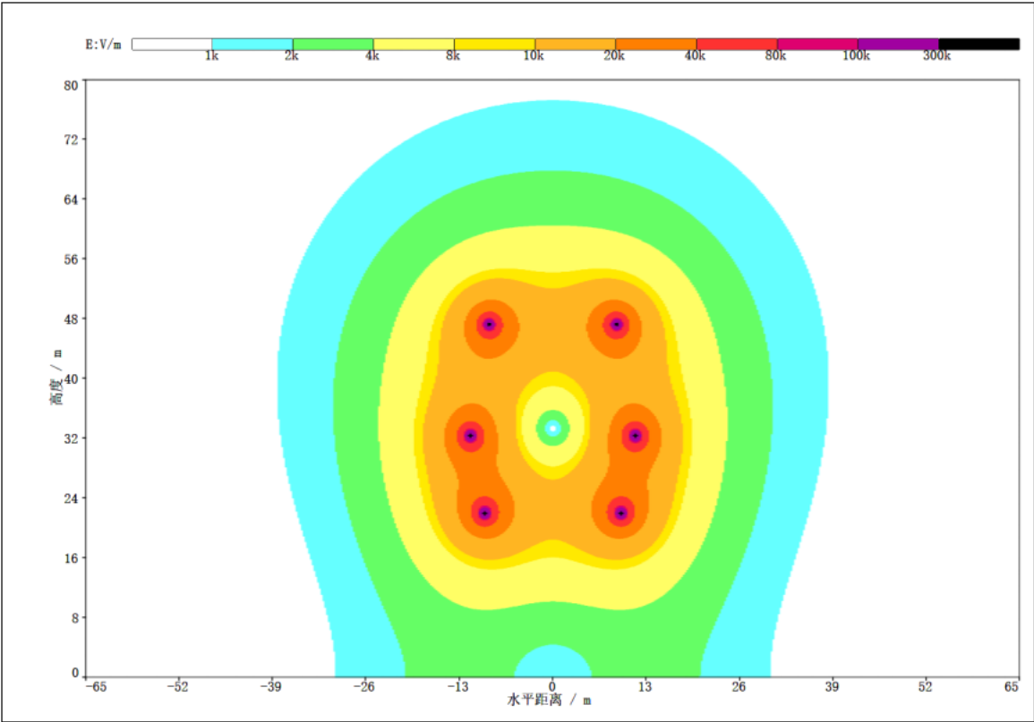
图 6.1-8 新建段 500kV 同塔双回线路 4kV/m 等值线分布图
