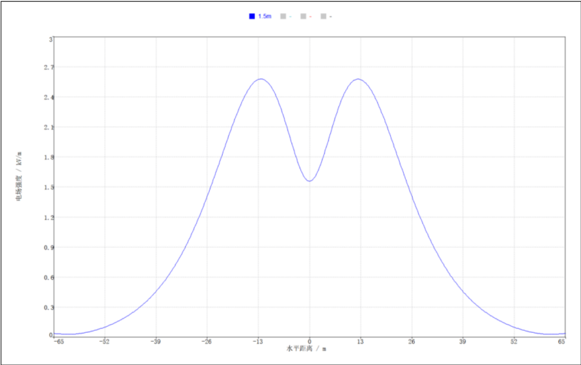
图 6.1-4 新建段 500kV 同塔双回线路工频电场强度分布曲线图
