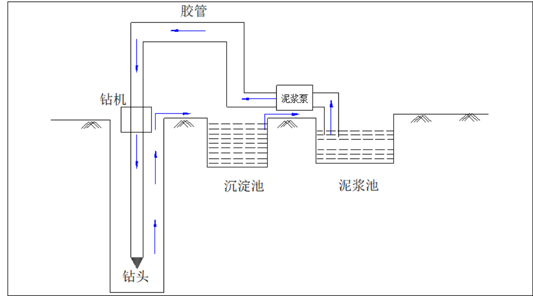
图 3.1-5 采用泥浆护壁钻机反循环法钻进施工工艺
