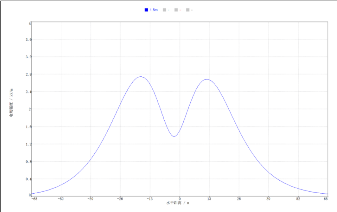
图 6.1-2 恢复架线段 500kV 同塔双回线路工频电场强度分布曲线图
