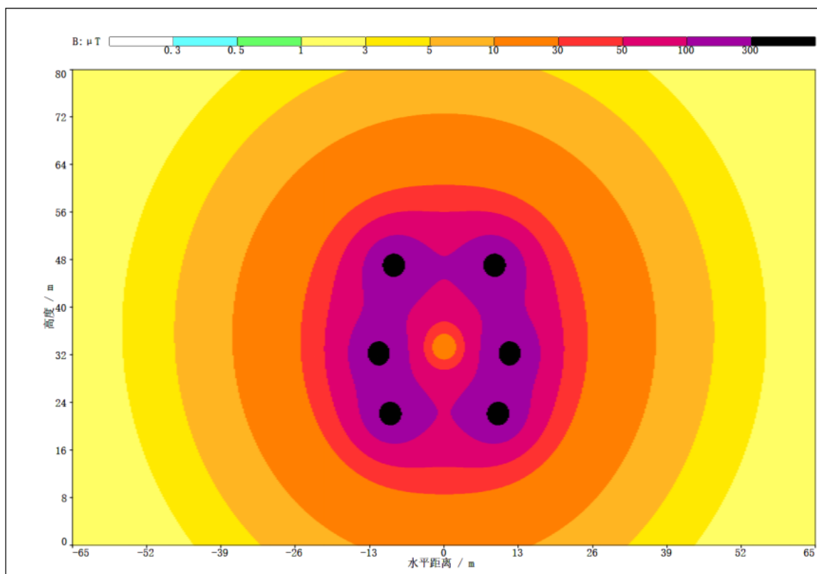
图 6.1-9 新建段 500kV 同塔双回线路 100 \mu T 等值线分布图
