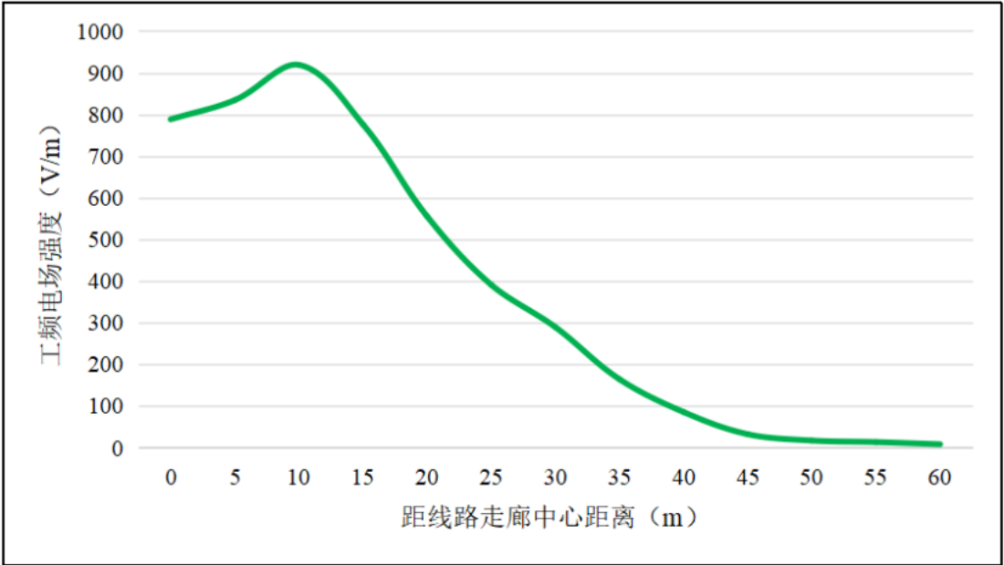
图 6.1-1 类比线路工频电场强度变化趋势示意图
