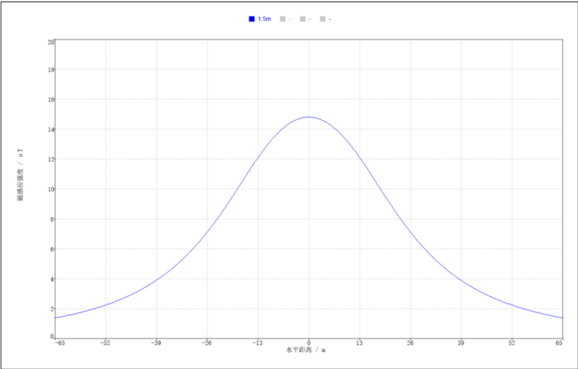
图 6.1-5 新建段 500kV 同塔双回线路工频磁感应强度分布曲线图
