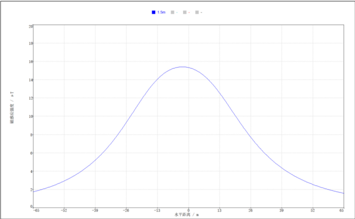
图 6.1-3 恢复架线段 500kV 同塔双回线路工频磁感应强度分布曲线图
