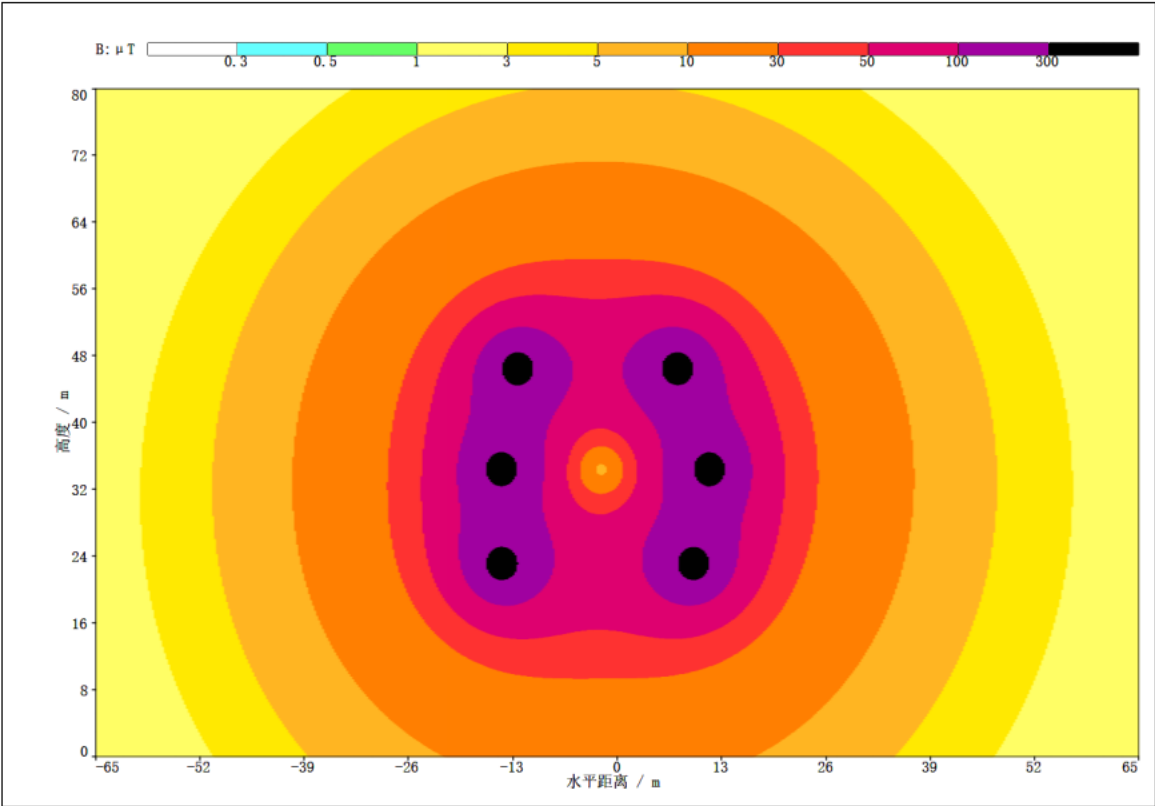
图 6.1-7 恢复架线段 500kV 同塔双回线路 100 \mu\text{T} 等值线分布图
