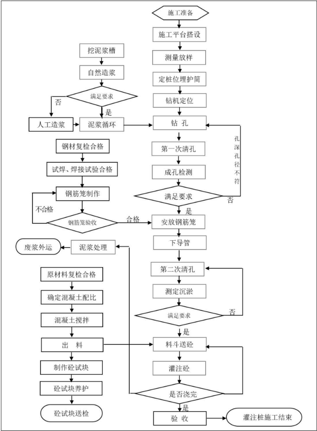
图 3.1-3 钻孔灌注桩的施工程序图
