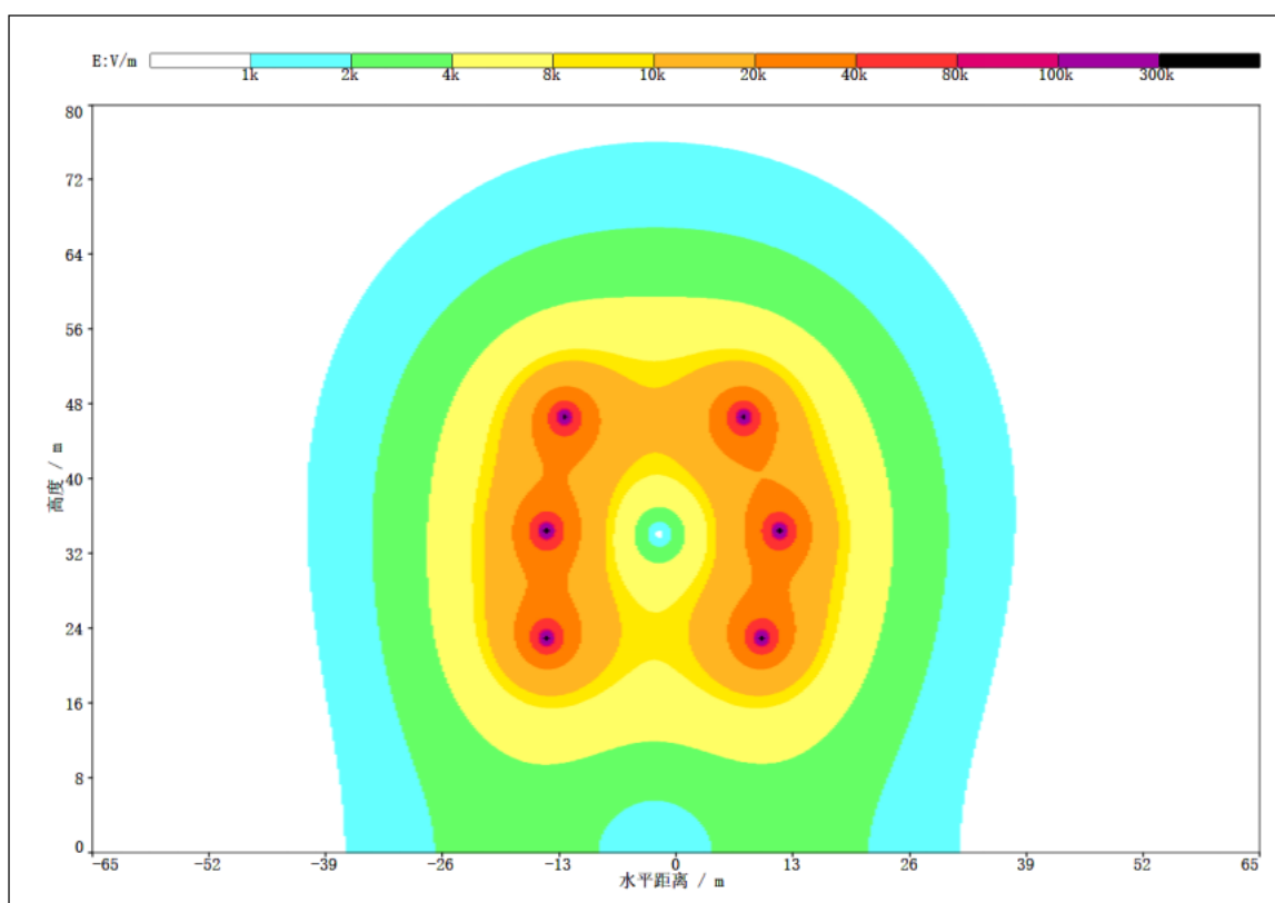
图 6.1-6 恢复架线段 500kV 同塔双回线路 4kV/m 等值线分布图
