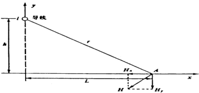
图6.1-1 磁场向量图
