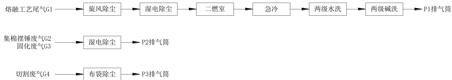
图 6.1-1 有组织废气处理示意图
