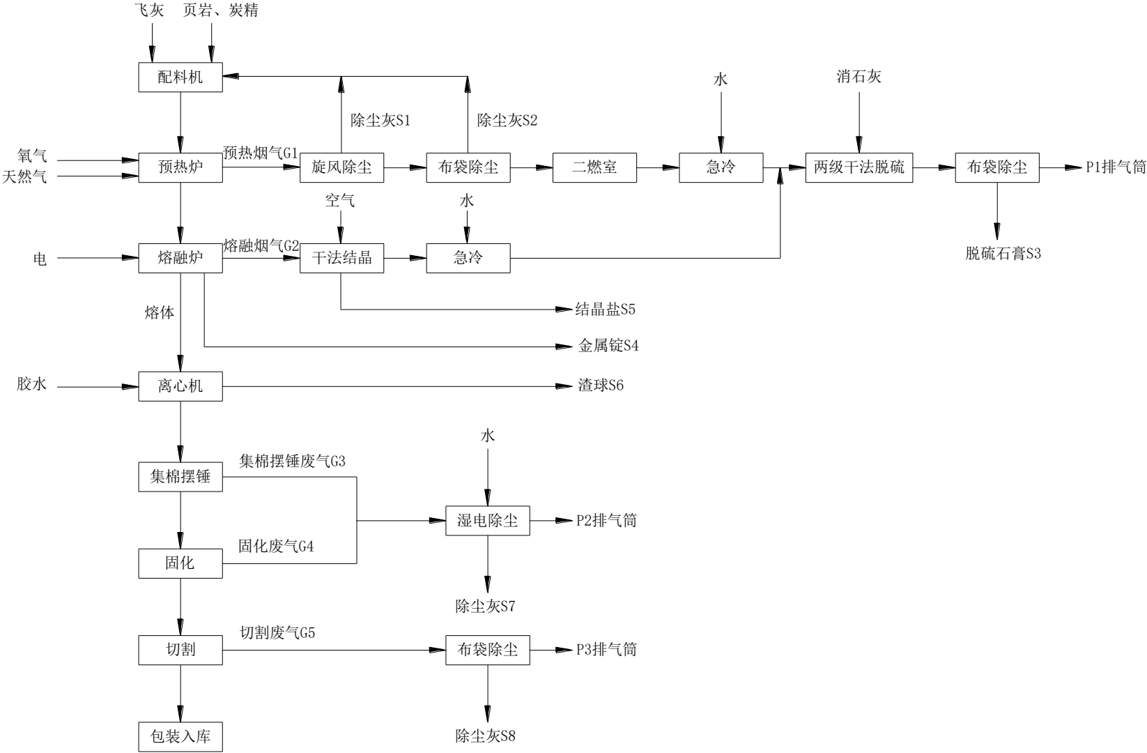
图 3.2-1 工艺流程图
