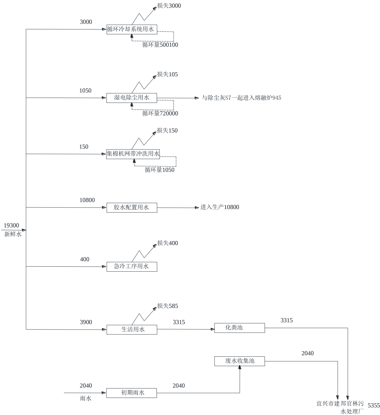
图 3.4-1 本项目水平衡（单位：t/a）
